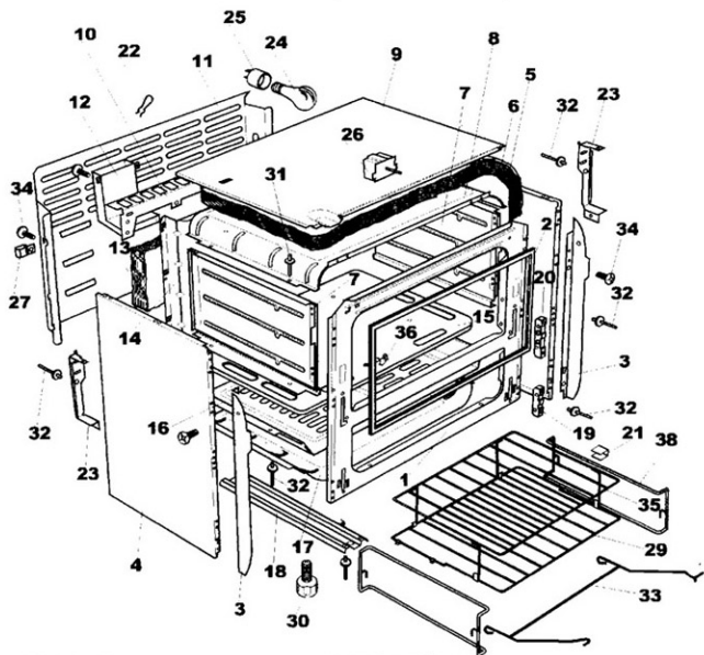
MODELOS GRILL
