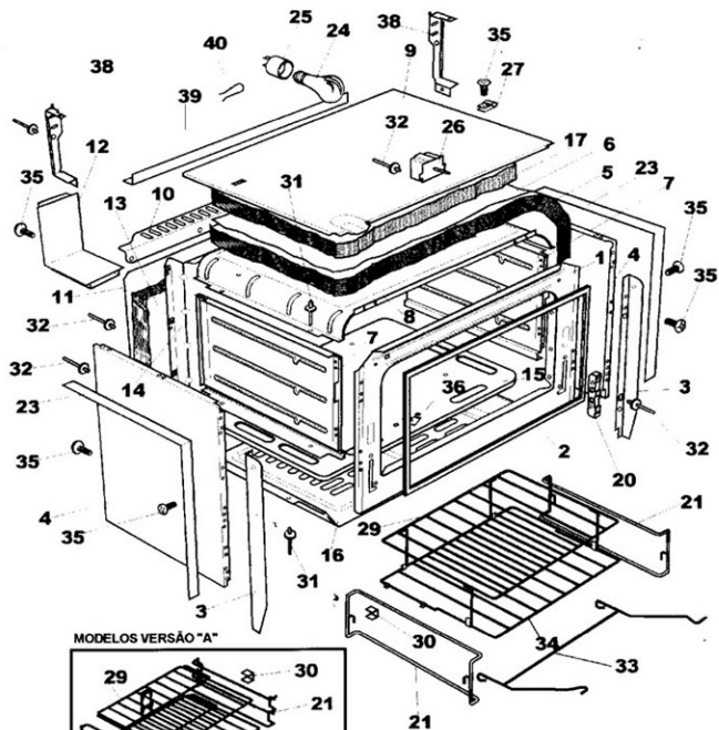
MODELOS GRILL
