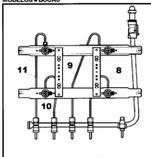
MODELOS 4 BOCAS
