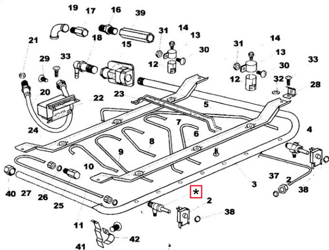
MODELOS 4 BOCAS
